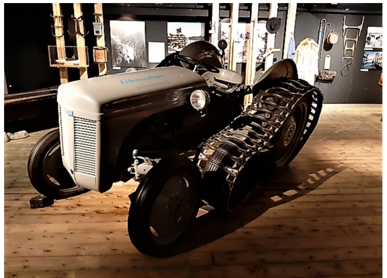
En Gråtass (Ferguson TE20) med belter ble brukt i skogen.
